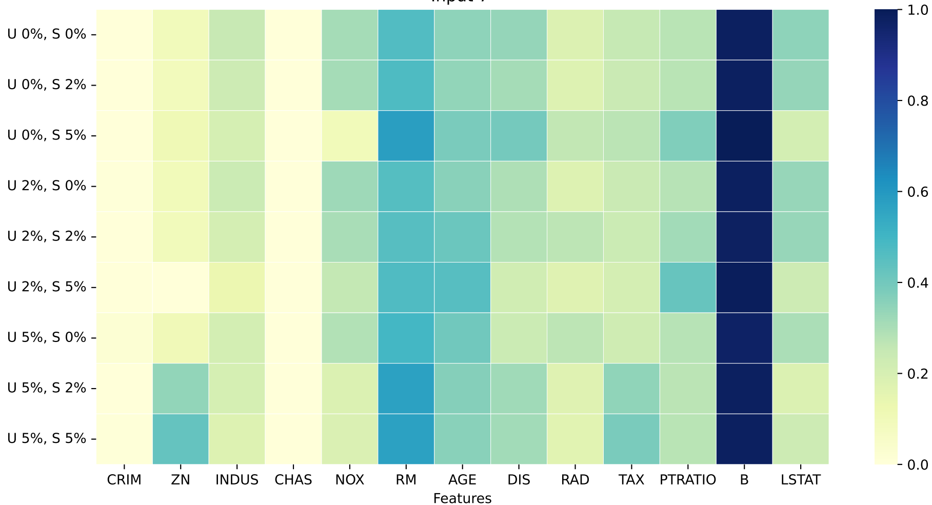
Input 7
